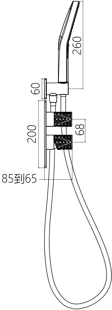
左视图
