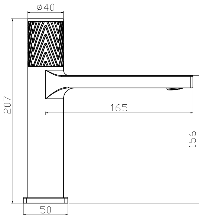
左视图
